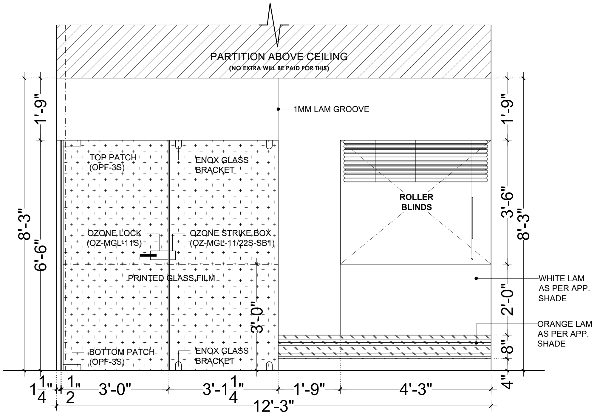
ELEVATION (PT2)
