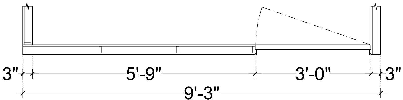
PLAN (PT8)
