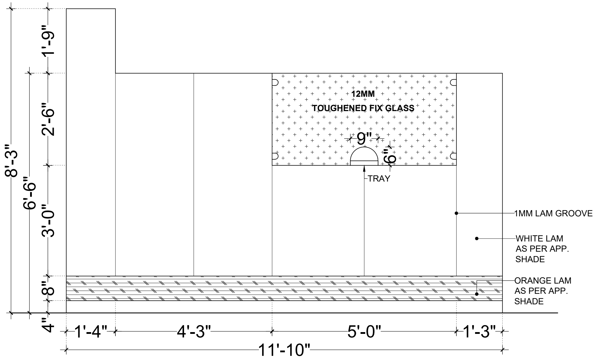
ELEVATION (PT3)
