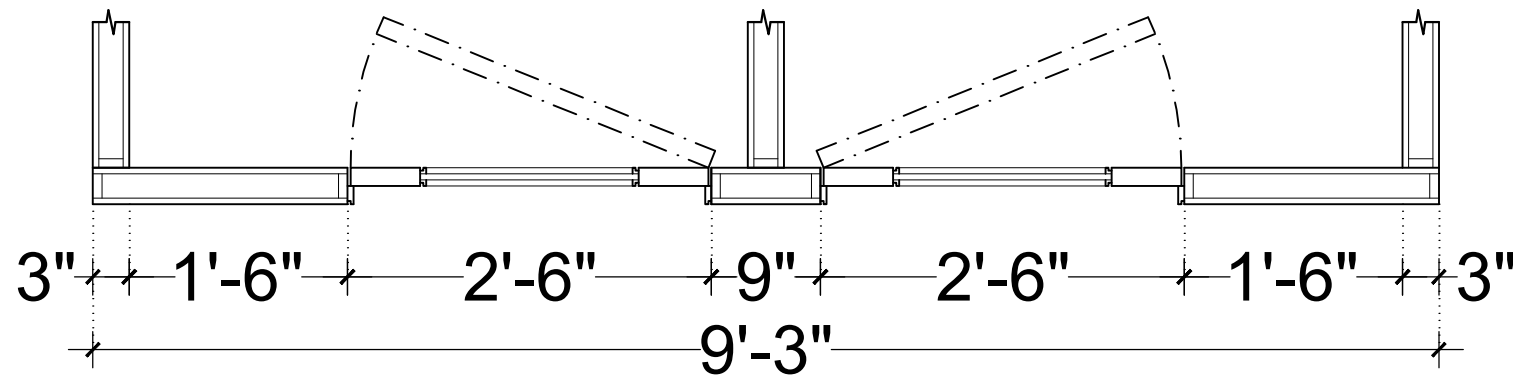
PLAN (PT6)
