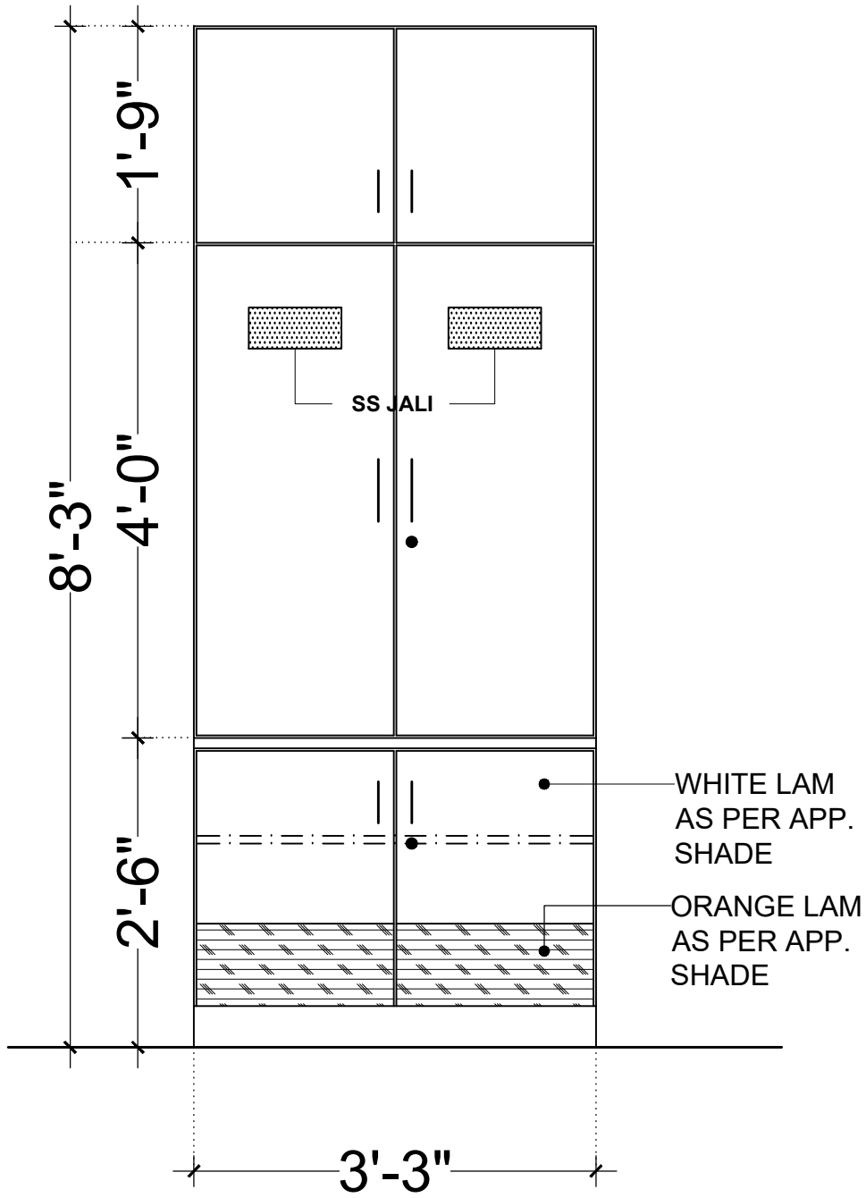
ELEVATION (CB6)
