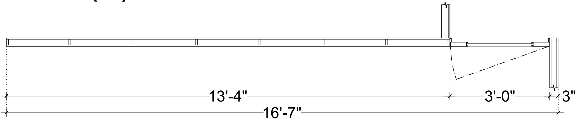
ELEVATION (PT7)
