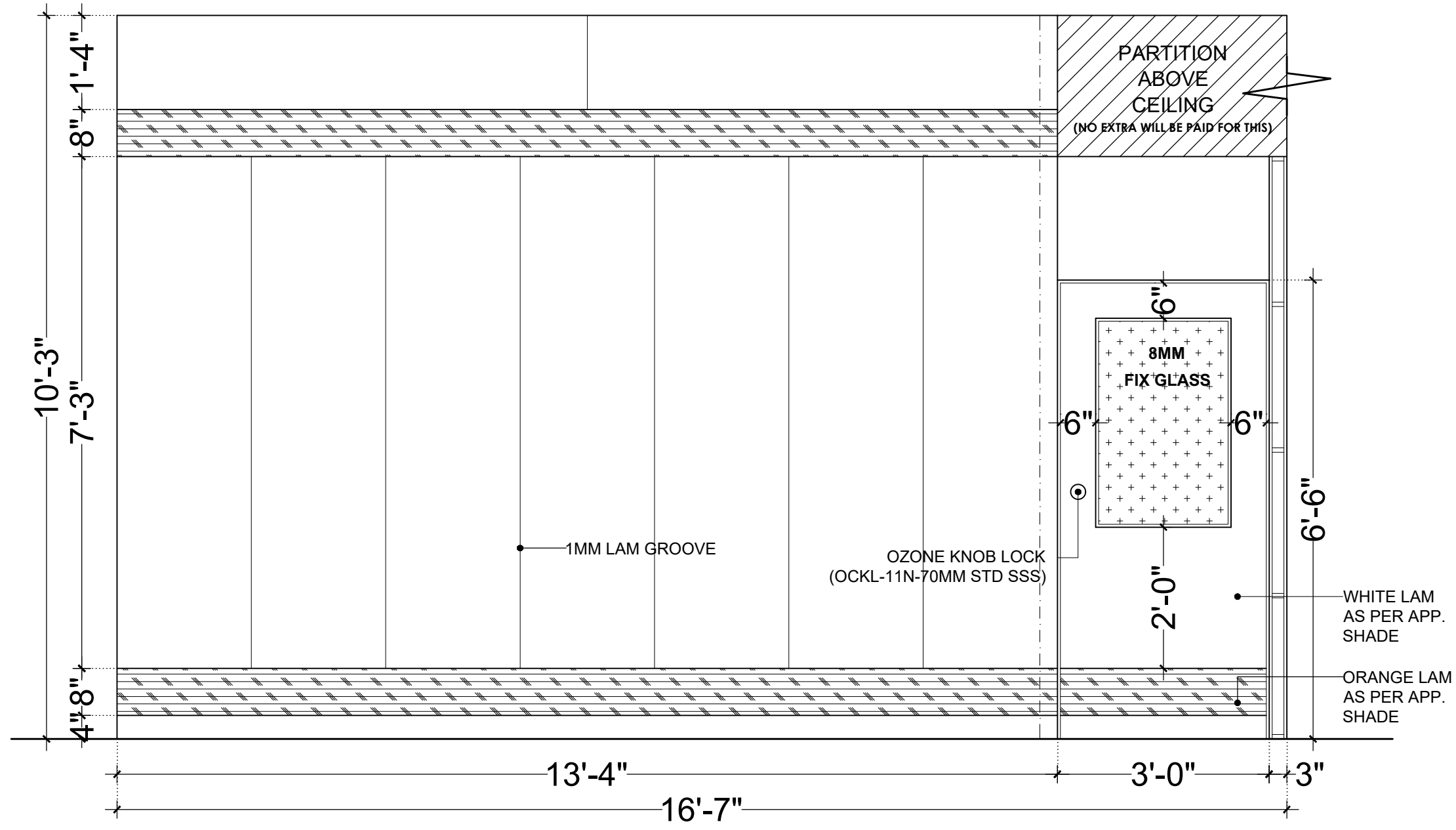
ELEVATION (PT7)
